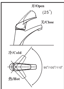
单把手产品/One handle
